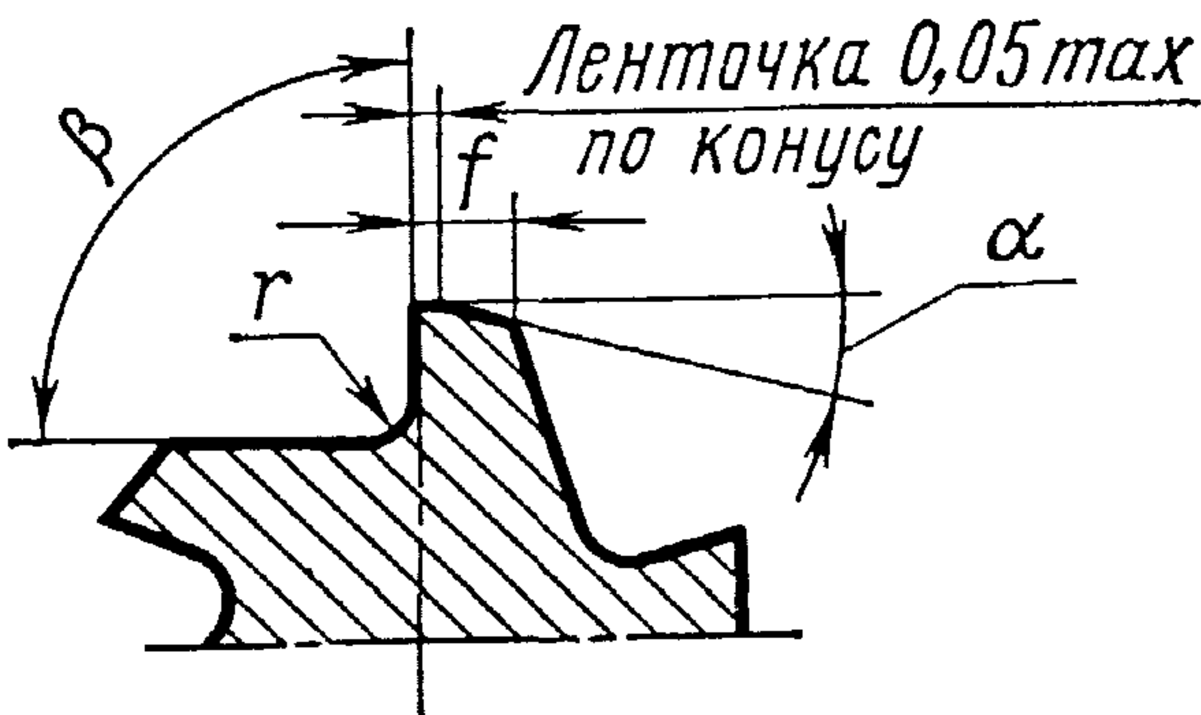
Размеры в мм
